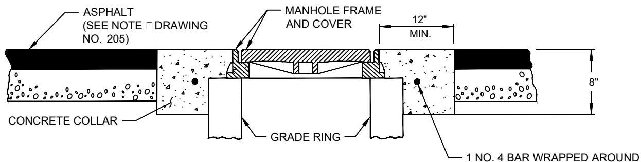
SECTION A-A
