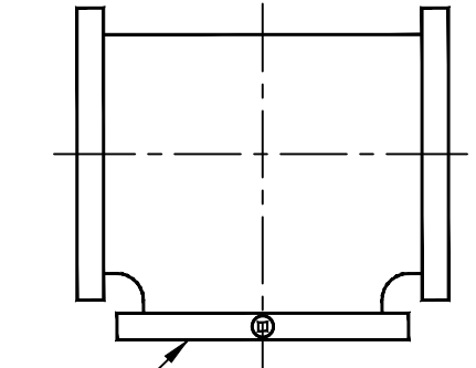
TEE
