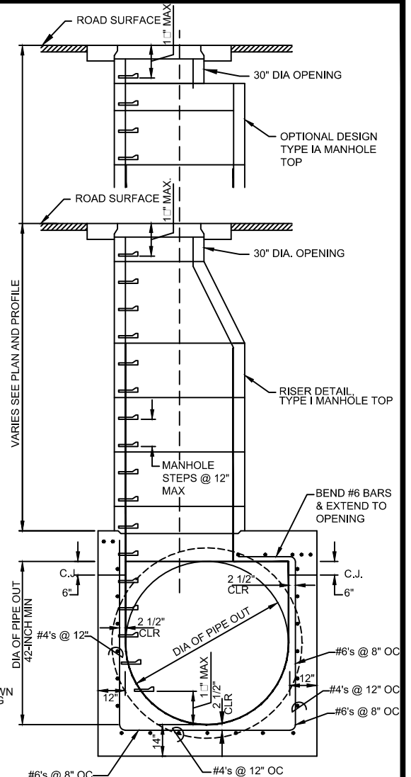
SECTION A-A
